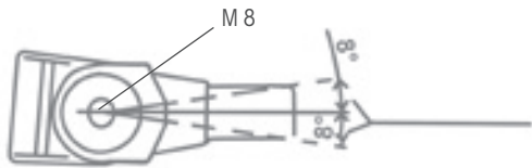
Schnitt durch das Drehgelenk (oberes Rohrverbindungsstück)
